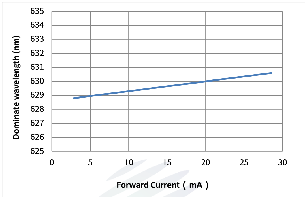
Fig. 1-12 Forward current VS Dominant wavelength 正向电流与主波长特性曲线 (Ts=25°C)
