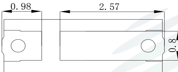
Fig.1-3 Bottom view 背面视图
