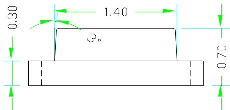
侧面视图
