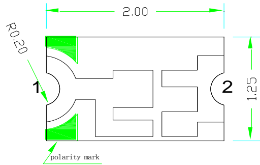
正面视图
